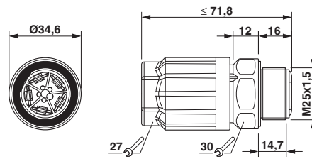
Maßzeichnung
