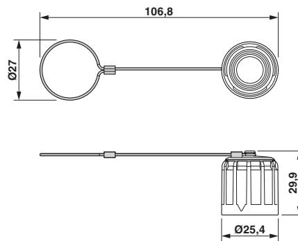
Maßzeichnung
