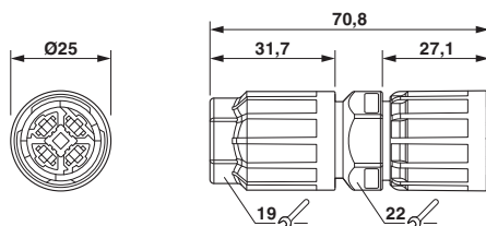
Maßzeichnung
