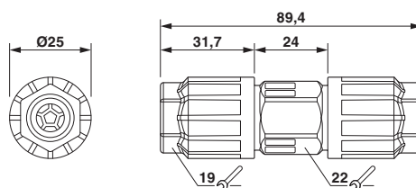
Maßzeichnung
