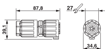
Maßbild: Steckverbinder, 2,5 mm 2
